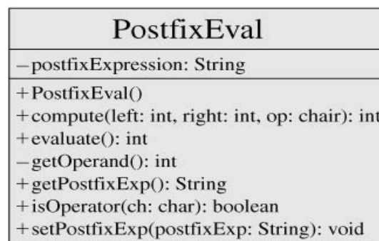
Gambar 3. UML dari Class PostfixEval
