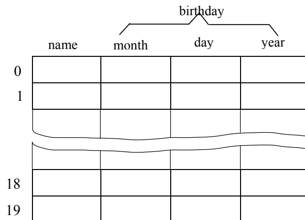
Gambar 9.4 Array dari struktur
